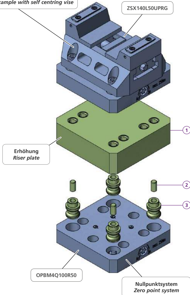
Anwendungsbeispiel mit Zentrischspanner Application example with self centring vise
