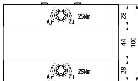
Anwendungsbeispiel mit Zentrischspanner Application example with self centring vise
