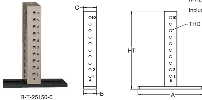
R-T-25150-6
