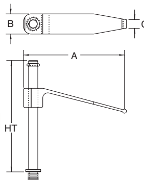
R-CT-64-70-6 R-CT-40-30-6
